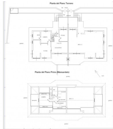
PLANIMETRIA INDICATIVA
