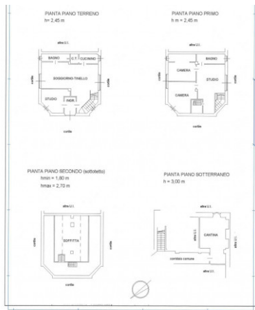
PLANIMETRIA INDICATIVA
