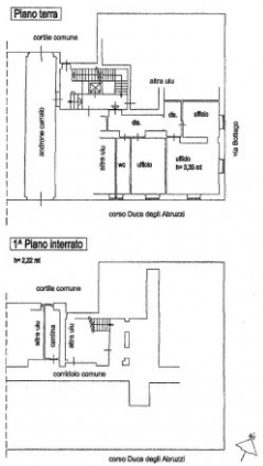
PLANIMETRIA INDICATIVA
