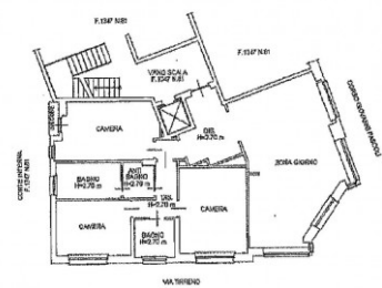
PLANIMETRIA INDICATIVA
