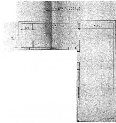
PLANIMETRIA INDICATIVA
