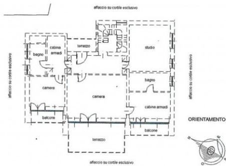
PIANTA PIANO PRIMO - H. 3.00 mt
