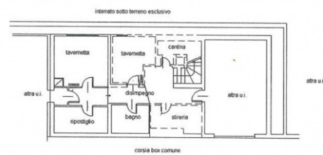
PIANTA PIANO INTERRATO - H. 2.50 mt
