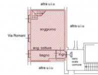
PIANTA PIANO SECONDO (3° f.t.) h = 3,30
