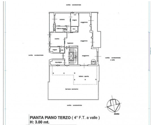
PLANIMETRIA INDICATIVA
