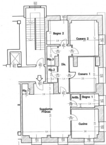
piano secondo - appartamento scala 1:100
